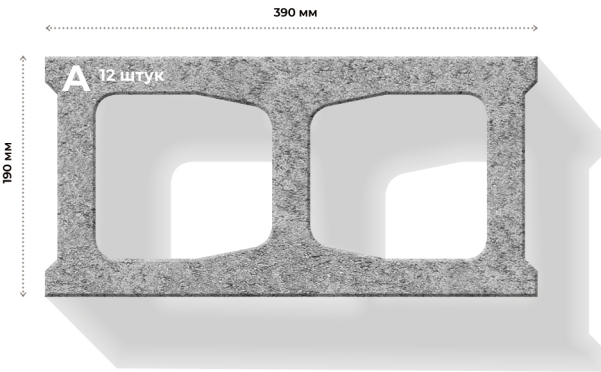
Розміри елементів та їх кількість в ряді
